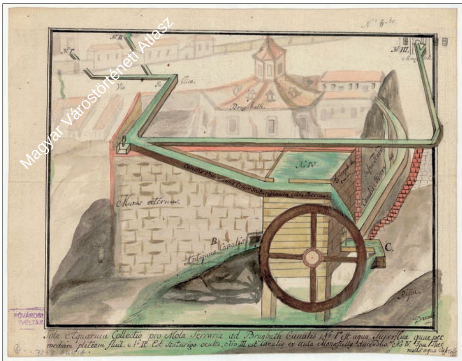
69. ábra. Fűrészmalom terve a Rudas fürdőnél, 18. század közepe Budapest Főváros Levéltára BFL XV.17.a.302 No. 140 a, f Fig. 69 Plan of sawmill at Rudas Baths, middle of the 18th century Budapest City Archives BFL XV.17.a.302 No. 140 a, f
