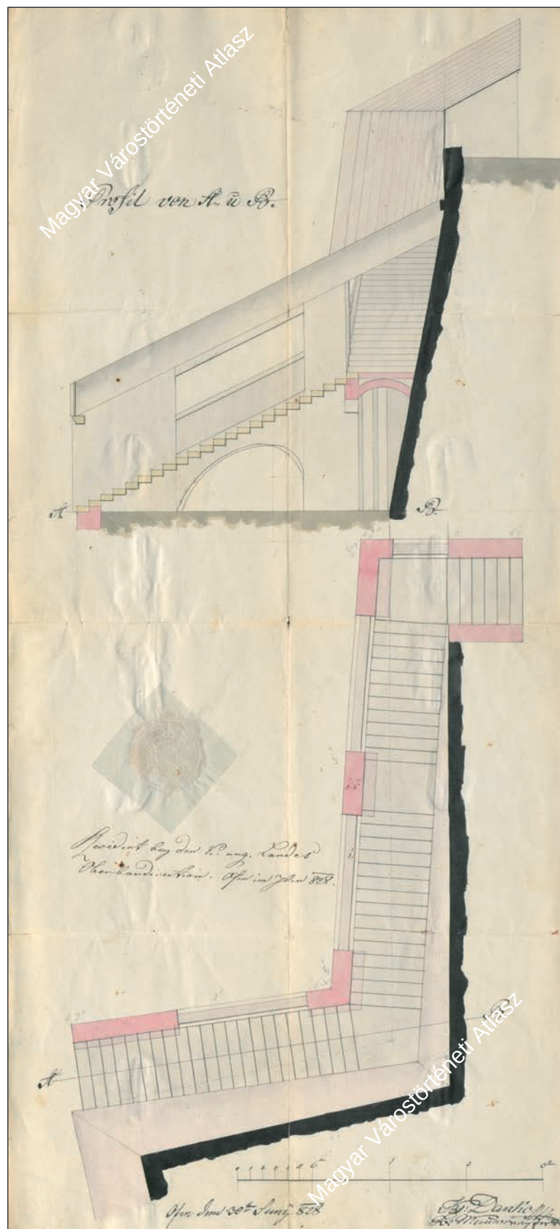
67. ábra. Dankó József: a Várba vezető lépcső (Nándor-lépcső), 1828 Budapest Főváros Levéltára BFL XV.17.a.303/165a Fig. 67 József Dankó: stairway to the Castle (Nándor stairs), 1828 Budapest City Archives BFL XV.17.a.303/165a
