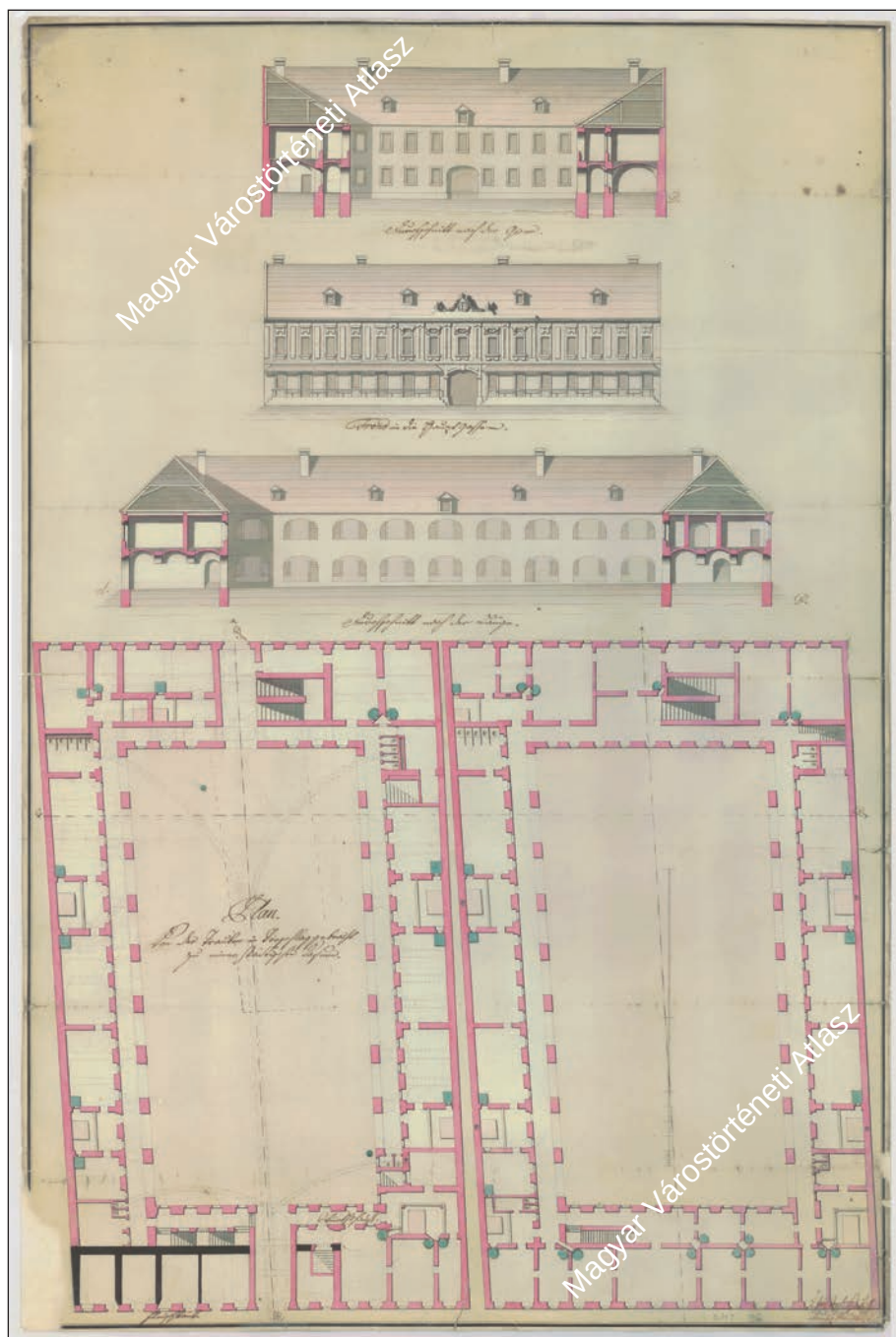
48. ábra. Hickisch Kristóf: A Három Nyúl kaszárnya terve, 1792 Budapest Főváros Levéltára BFL XV.17.a.302/96 Fig. 48 Kristóf Hickisch: Plan of the Three Rabbits Barracks, 1792 Budapest City Archives BFL XV.17.a.302/96
