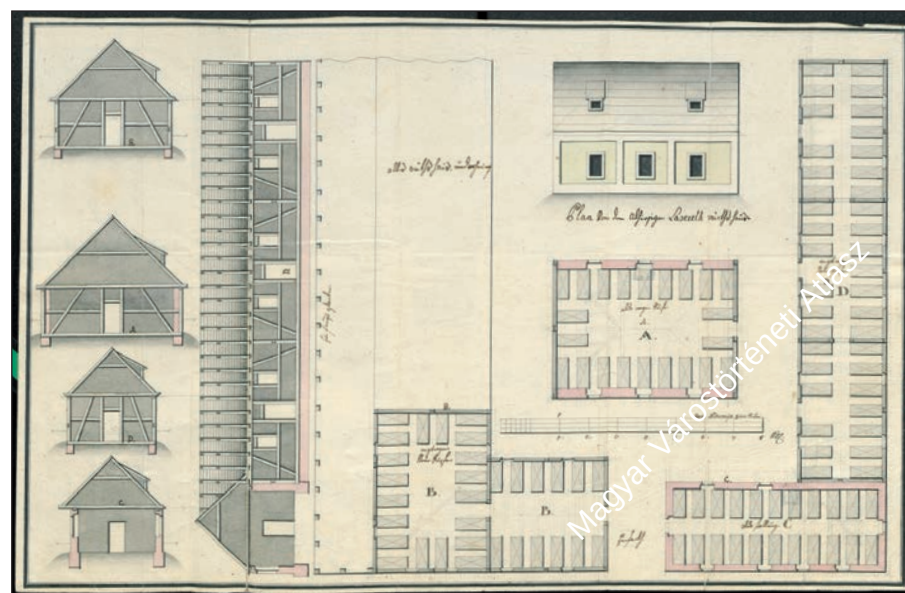
54. ábra. Reischl János Gáspár: az ún. Lazarérum-fogadó (Lazareth Wirtshaus), 1789 Budapest Főváros Levéltára BFL XV.17.a.303/192a-b Fig. 54 János Gáspár Reischl: the so-called Lazareth Inn (Lazareth Wirtshaus), 1789 Budapest City Archives BFL XV.17.a.303/192a-b
