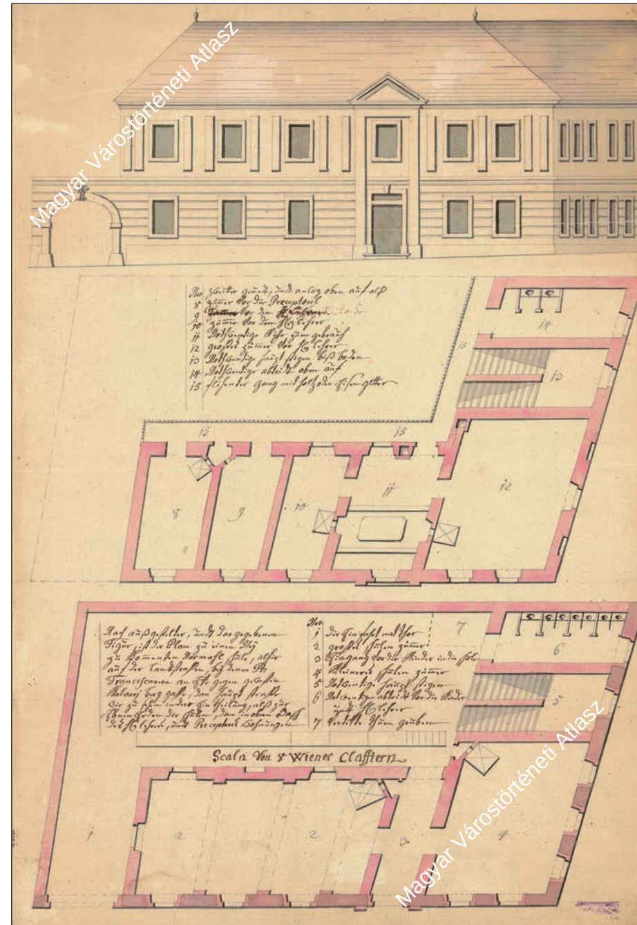
58. ábra. Az országúti elemi iskola terve, 1794 Budapest Főváros Levéltára BFL XV.17.a.302 No. 100 Fig. 58 Plan of the elementary school in Országút, 1794 Budapest City Archives BFL XV.17.a.302 No. 100
