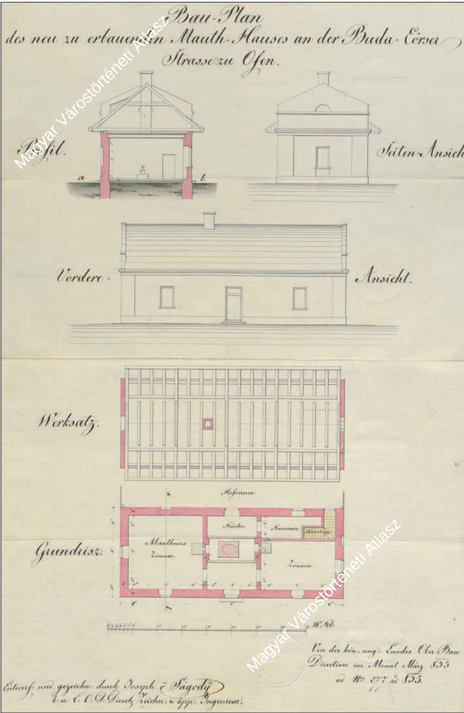
52. ábra. Ságody József: a mai Budaörsi úti vámház terve, 1835 Budapest Főváros Levéltára BFL XV.17.a.303/166a Fig. 52 József Ságody: Plan of tollhouse in modern Budaörsi Road, 1835 Budapest City Archive BFL XV.17.a.303/166a
