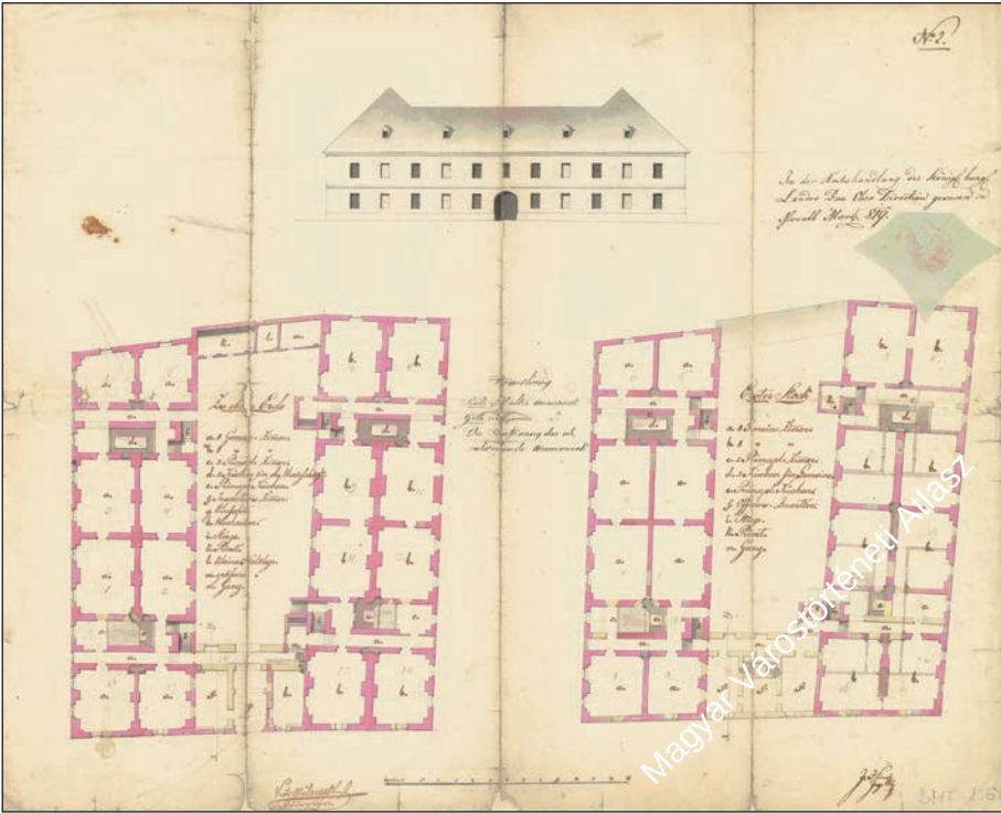
47. ábra. A Császárrésnél álló kaszárnyák tervei Budapest Főváros Levéltára BFL XV.17.a.302 No. 156. Fig. 47 Plan of the barracks at the Kaiser's Gap Budapest City Archive BFL XV.17.a.302 No. 156
