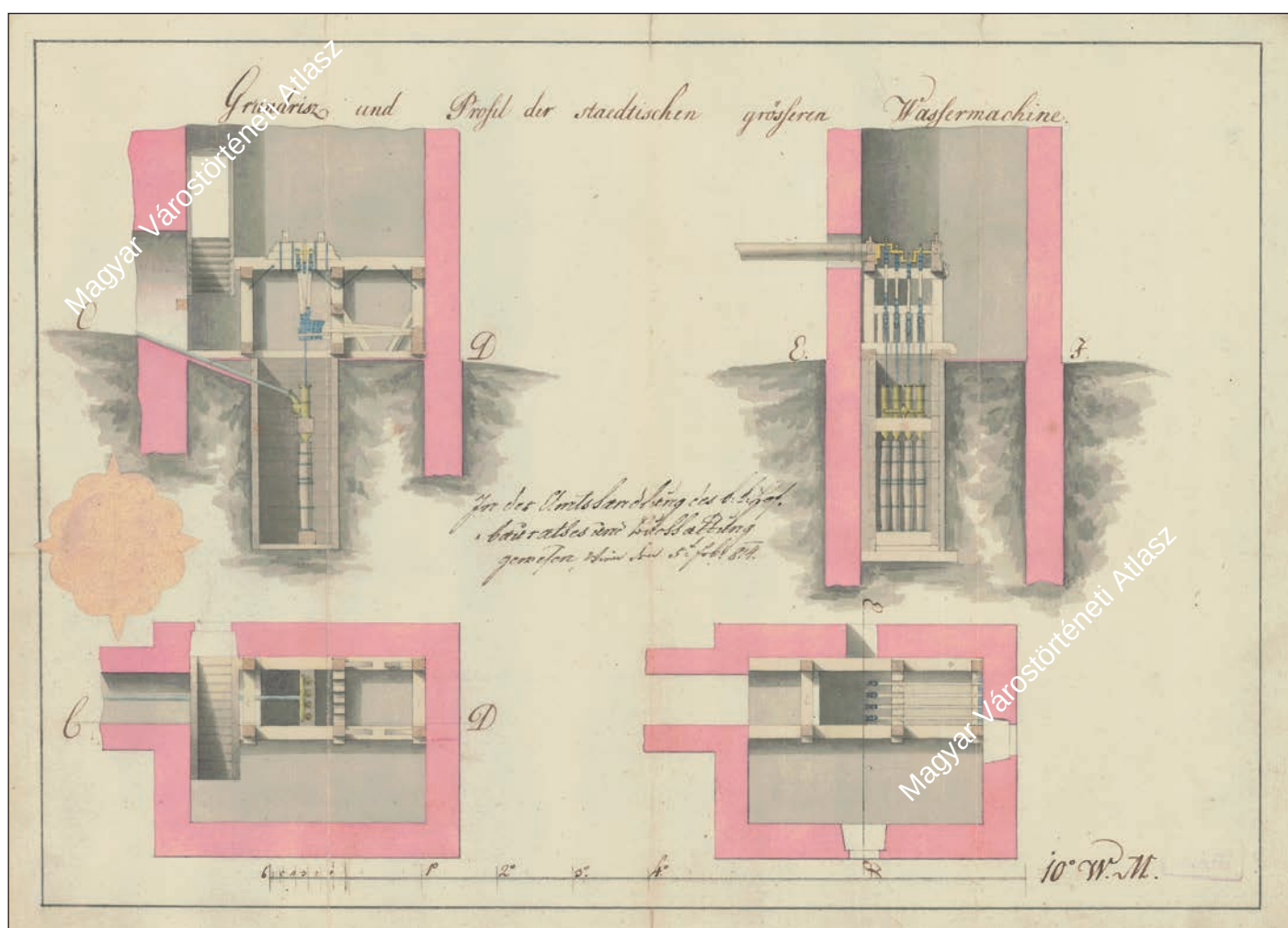
64. ábra. Dunai vízmű terve, 1814 Budapest Főváros Levéltára BFL XV.17.a.302 No. 145 Fig. 64 Plan of the Danubian waterwork, 1814 Budapest City Archives BFL XV.17.a.302 No. 145
