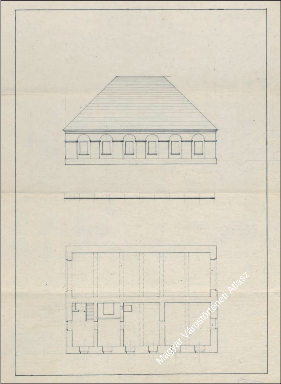
51. ábra. Az egykori tabáni sörház tervrajza, 1816 körül Budapest Főváros Levéltára BFL XV.17.a.303/187 Fig. 51 Plan of the former beerhouse in Tabán, around 1816 Budapest City Archives BFL XV.17.a.303/187)
