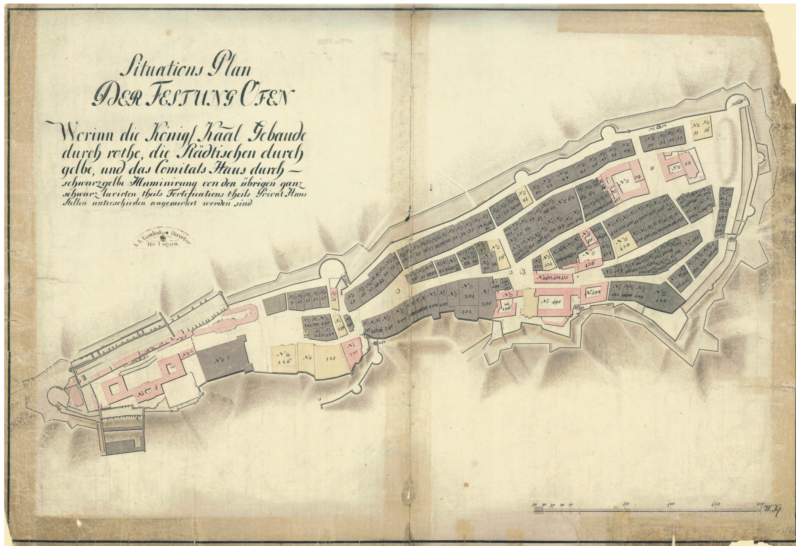
C.1.5 A budai Vár helyszínrajza, 1786–1794 (BFL XV.16.a.203/2)
