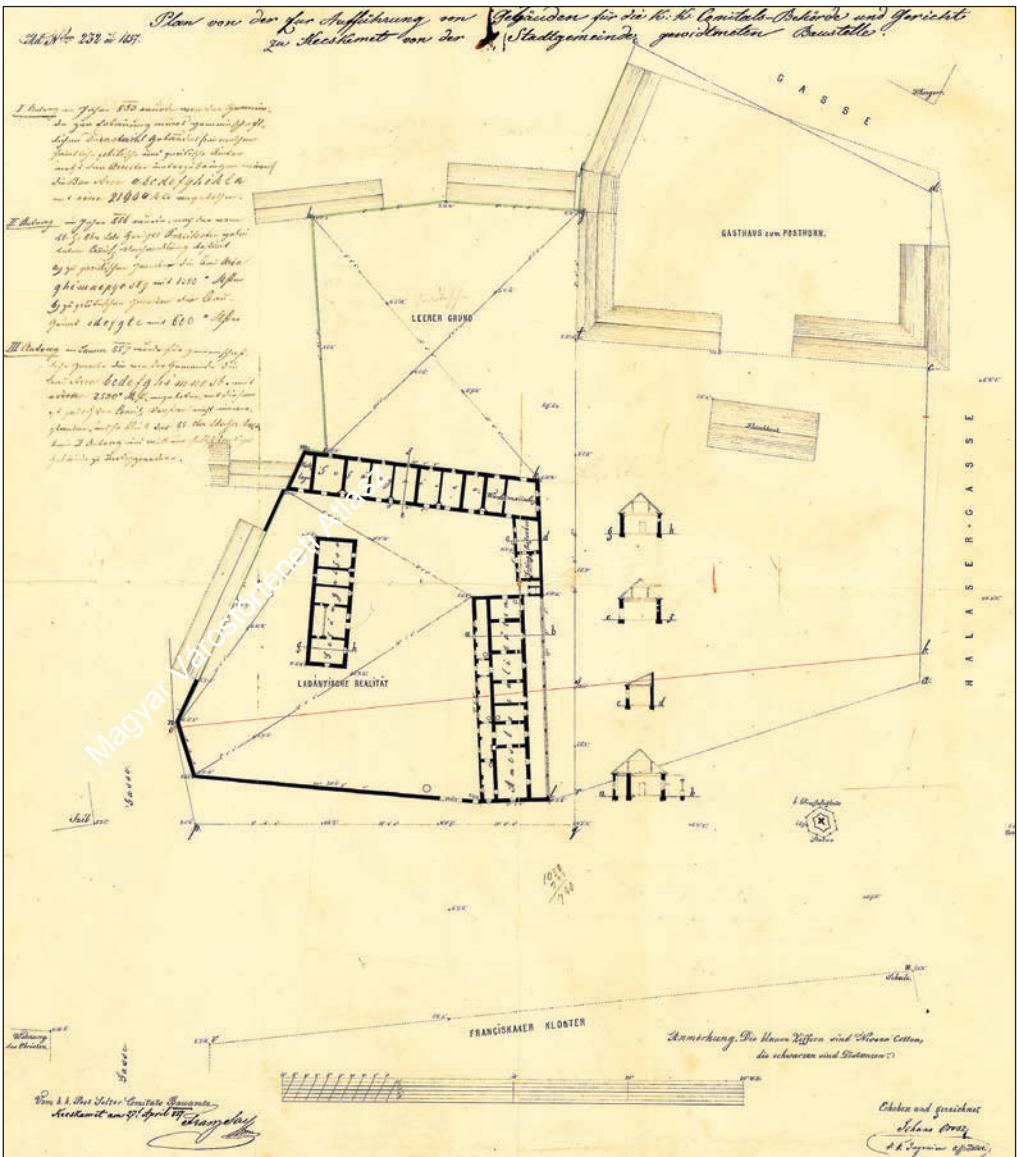
65. ábra. Az ún. Ladányi–Millhoffer ház tervei. Orosz, Johann Sach Ferenc: Plan von der zur Aufführung von Gebäuden für die k. k. Comitats-Behörde und Gericht zu Kecskemét von der Stadtgemeinde gewidmeten Baustelle. (A kecskeméti cs. és kir. megyei hatóságok és bíróság épületei részére a város közönsége által rendelkezésre bocsátott építési telek térképe). 1857. Magyar Nemzeti Levéltár Országos Levéltára S 101 No. 0382 Fig. 65 Plans of the so-called Ladányi–Millhoffer House. Ferenc, Johann Sach Orosz: Plan von der zur Aufführung von Gebäuden für die k. k. Comitats-Behörde und Gericht zu Kecskemét von der Stadtgemeinde gewidmeten Baustelle. 1857. Hungarian National Archives, National Archives of Hungary S 101 No. 0382
