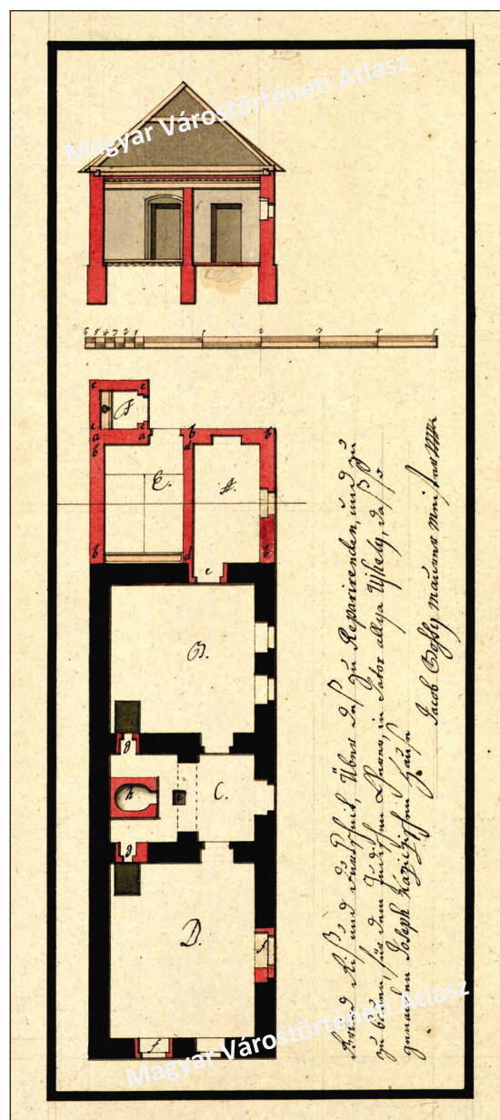
25. ábra. A zsidó tanító házána alaprajza 1792. (MOL T 62 1015.)
