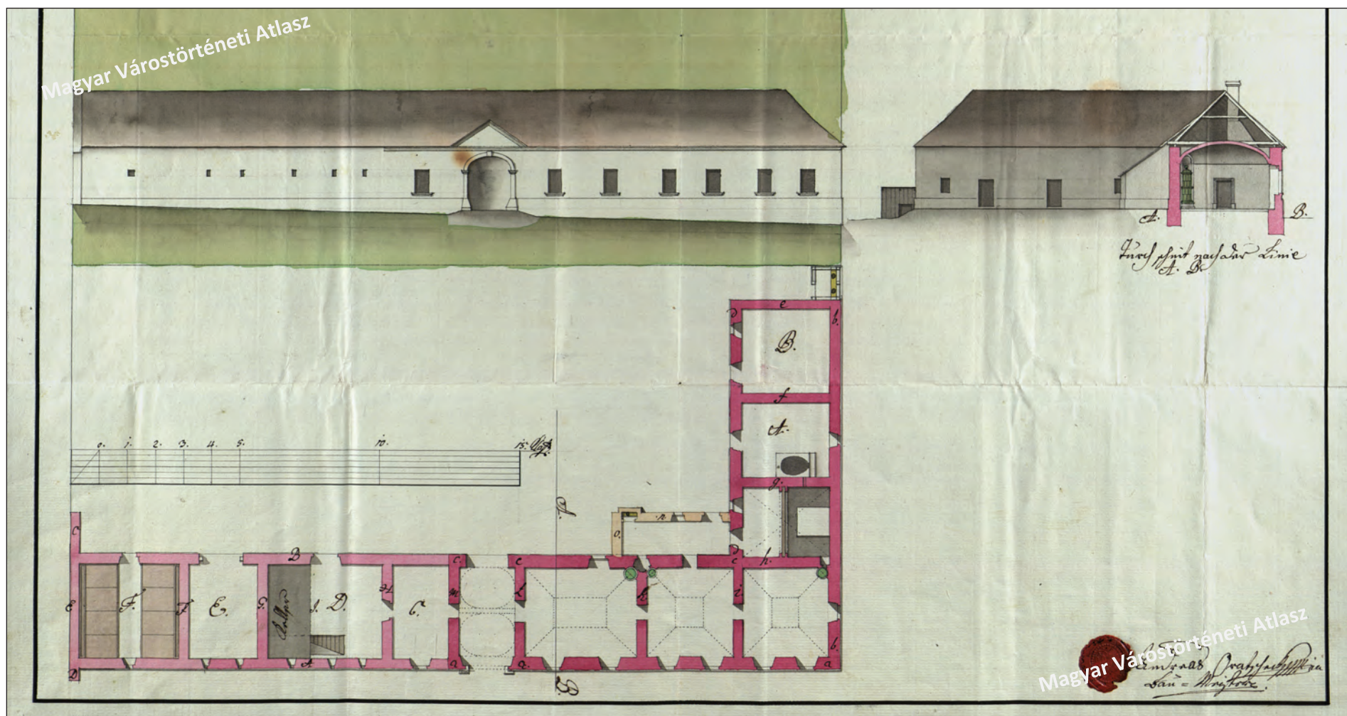
23. ábra. A Nedecki-ház alaprajza 1786. (MOL T62 1345) Fig. 23 Ground plan of the Nedecki house 1786 (MOL T62 1345)
