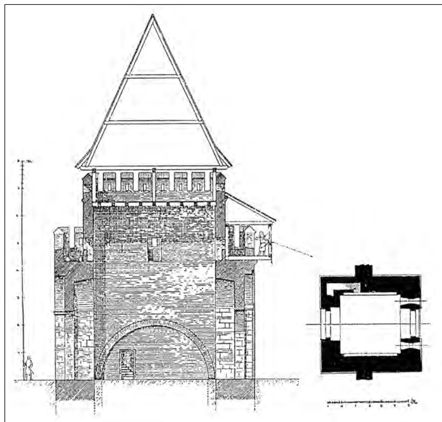
1. ábra: A déli kaputorony alaprajza és déli nézete (Cs. Sebestyén Károly rekonstrukciója)
