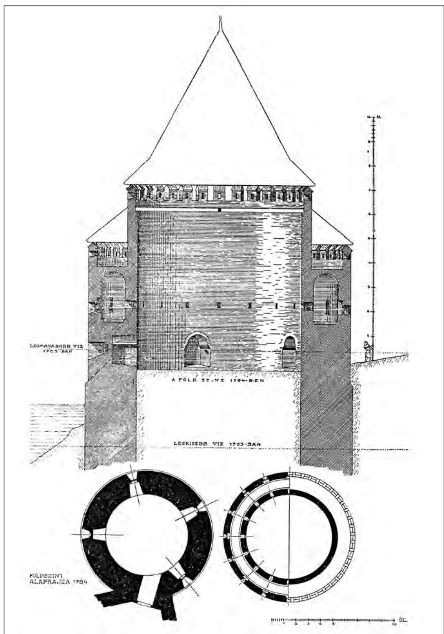
3. ábra: A vízitorony rekonstrukciója és vízszintes metszetei (Cs. Sebestyén Károly)
