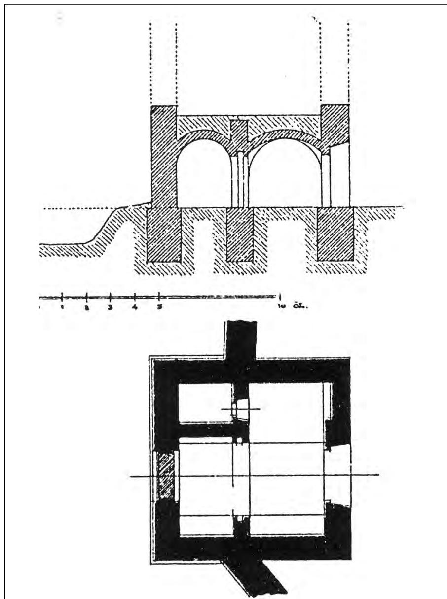
5. ábra: Az északi kaputorony alaprajza és metszete. Cs. Sebestyén Károly rekonstrukciója.
