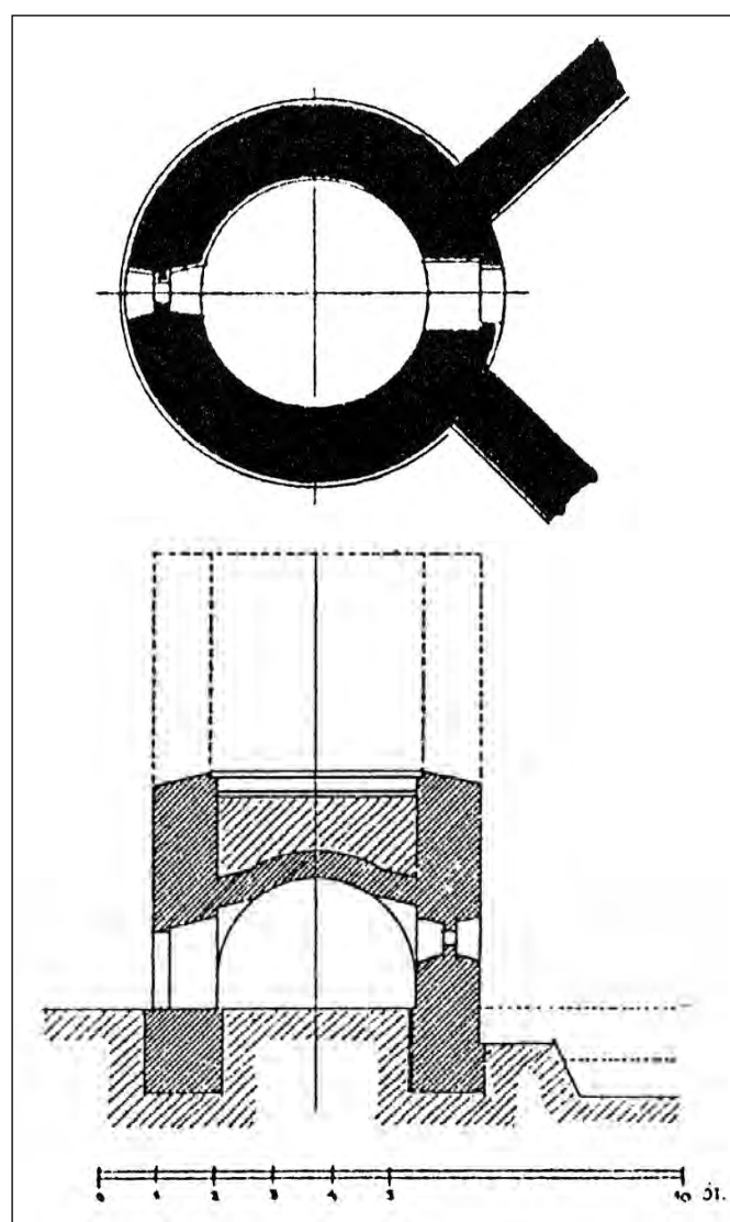
8. ábra: A délnyugati saroktorony alaprajza és metszete (Cs. Sebestyén Károly rekonstrukciója)
