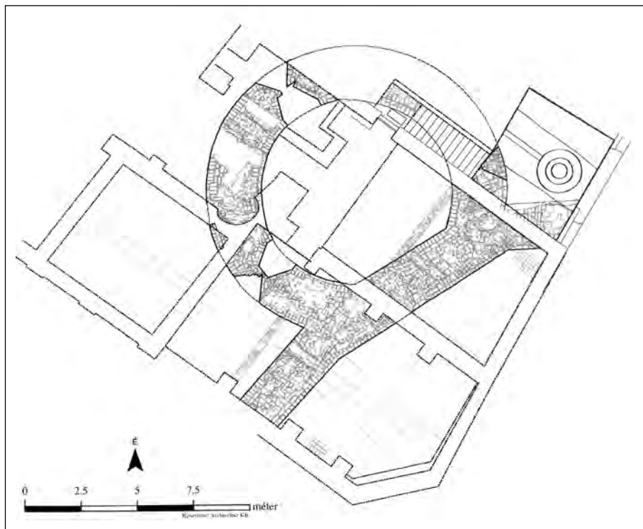
6. ábra: Az északnyugati saroktorony feltárt alaprajza (2007). Fogas Ottó felmérése
