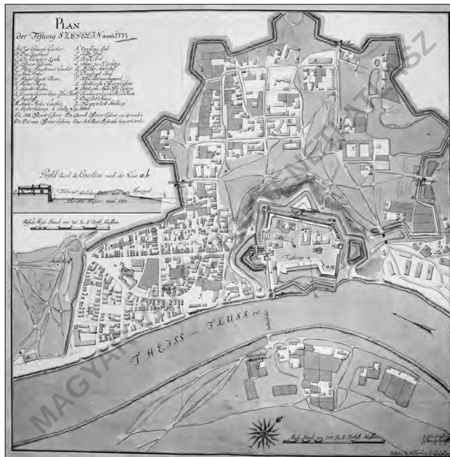
9. ábra: A Csillagsánc Wettstein von Westerheim felmérésén, 1774.
